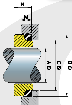
Dimensiones (Milímetros)
