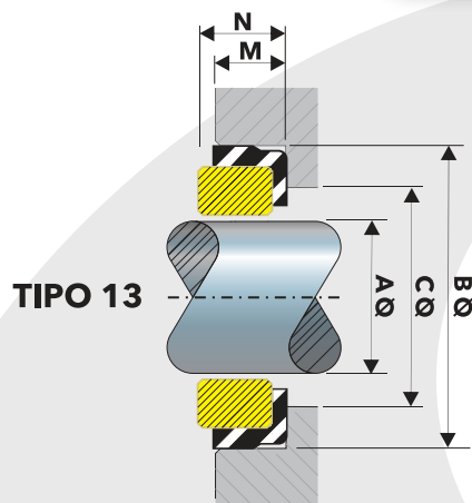
Dimensiones (Milímetros)
