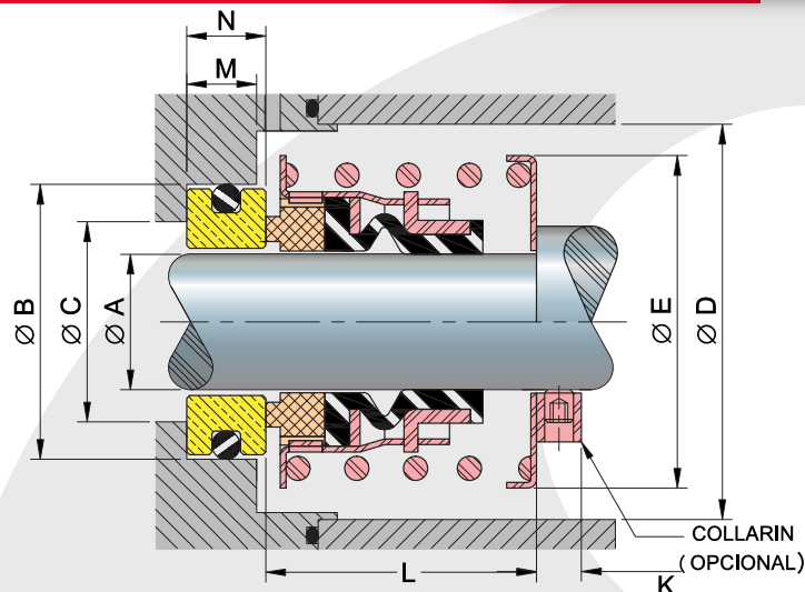
Dimensiones (Milímetros)
